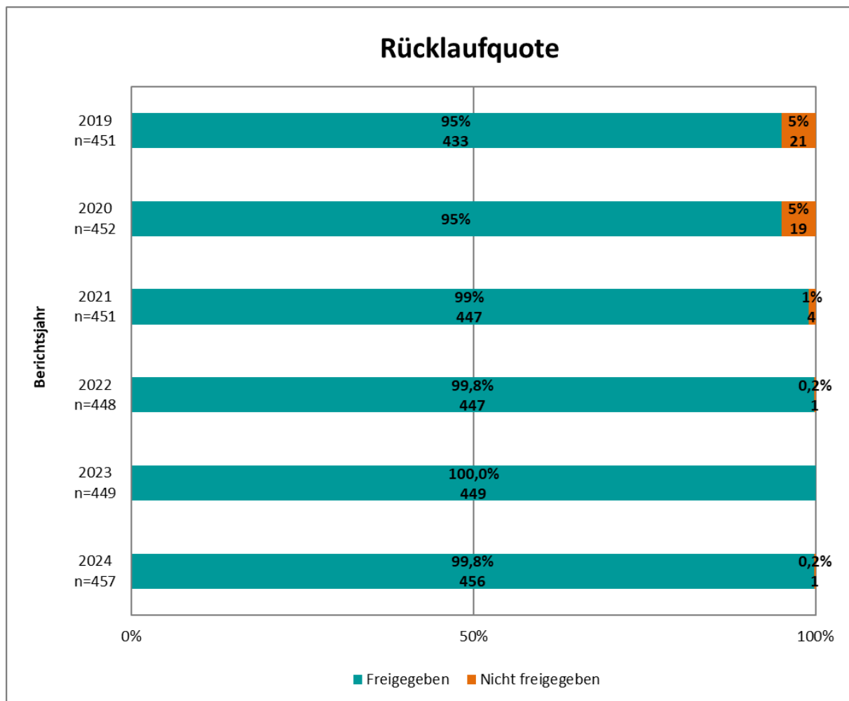
Abbildung 1: Rücklaufquote, Bj 2019 / 2020 / 2021 / 2022 / 2023 / 2024
