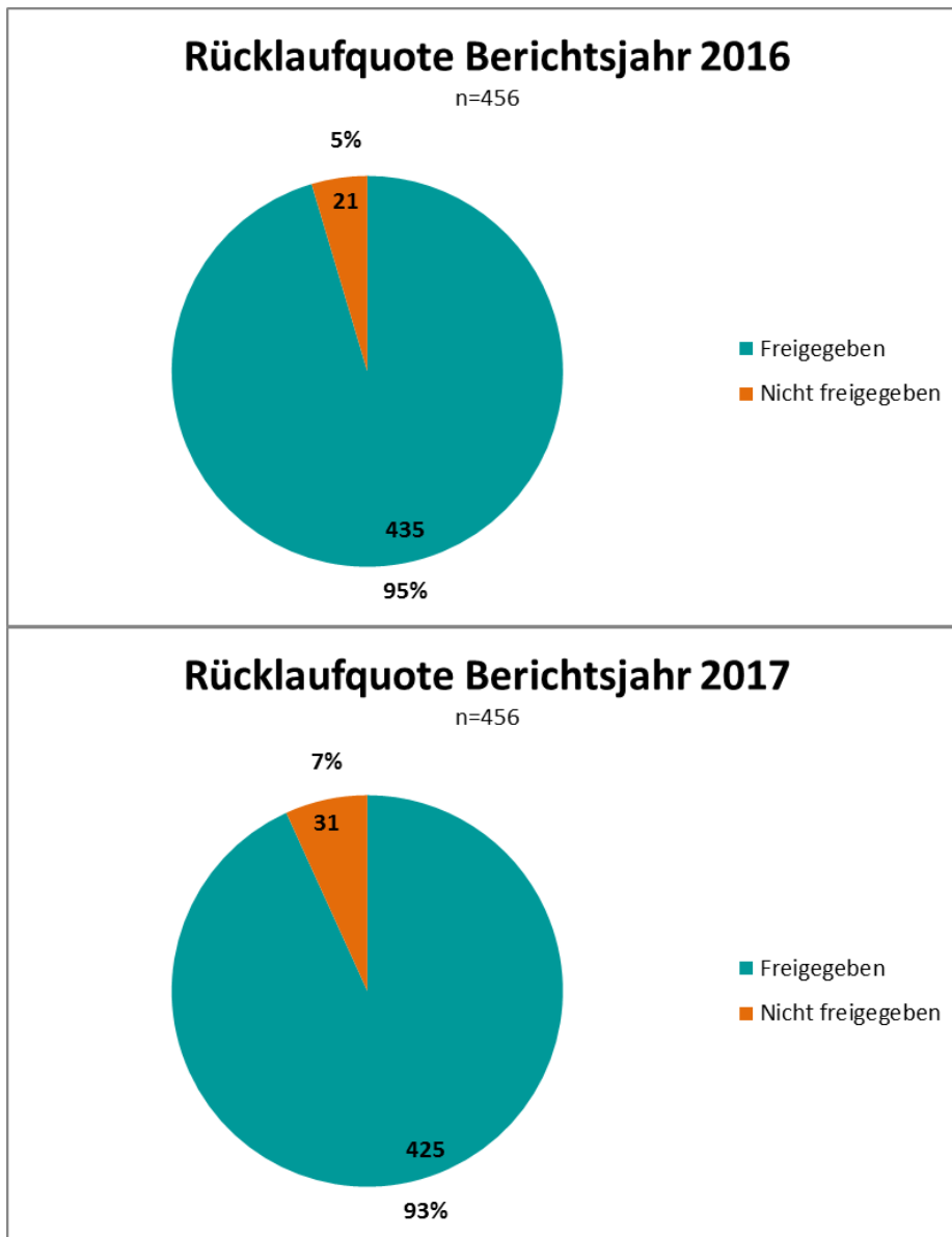
Abbildung 1: Rücklaufquote 8
